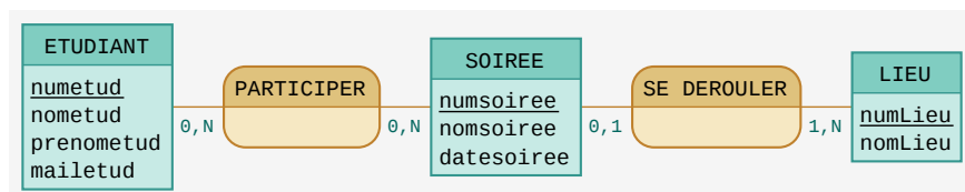
FIGURE 1.7 – Exemple cardinalités
